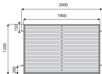
przęsło płotu
